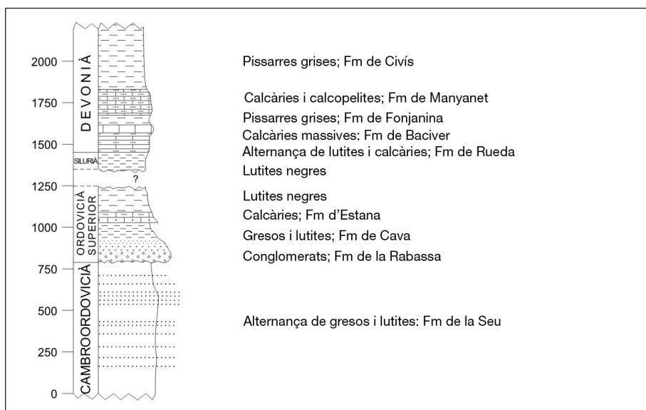
FIGURA 5. Columna estratigràfica sintètica dels materials sedimentaris paleozoics de la zona de les Planes de Son i la mata de València. Els gruixos dels diferents trams són orientatius; en aquesta àrea no és possible establir la potència dels sediments dels silurians.
