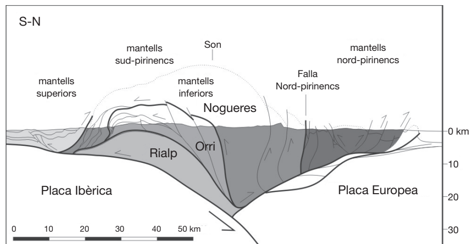
FIGURA 17. Tall geològic del conjunt dels mantells inferiors; de dalt a baix, són el mantell de Nogueres, el de l'Orri i el de Rialp. L'eix de l'Apilament Antiforme de la Zona Axial és al sud de la zona d'estudi, que se situa a tocar del límit nord del Mantell de l'Orri.
