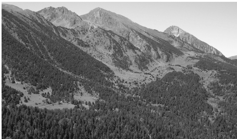
FIGURA 18. Lo Tésol vist des del pla de la Font. A les canals de lo Tonedor i les Estanyeres es reconeix la traça de l'estratificació dels carbonats devonians, cornianificats, molt redreçada. L'estructura interna del massís és obliqua a les pales, que tenen un pendent inferior i molt regular. Al peu de les pales es veu la morfologia característica de Campolado.
