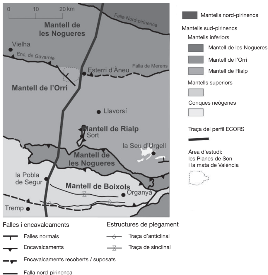
FIGURA 2. Esquema estructural de l'entorn de la zona d'estudi, indicada amb el requadre. Els Pirineus centrals formen part del conjunt dels mantells inferiors sud-pirínics. Aquests estan constituïts majoritàriament per roques sedimentàries, ígnies i metamòrfiques del Paleozoic. El registre sedimentari abraça des d'abans del Cambrià fins al Carbonífer (550 a 320 Ma) i, intruint en les roques sedimentàries, hi ha a més els batòlits hercinians que s'emporten al voltant del límit Carbonífer-Permian (300 Ma). La vall de Son i la mata de València se situen geològicament al Mantell de l'Orri i en el flanc nord de l'Apilament Antiforme de la Zona Axial.
