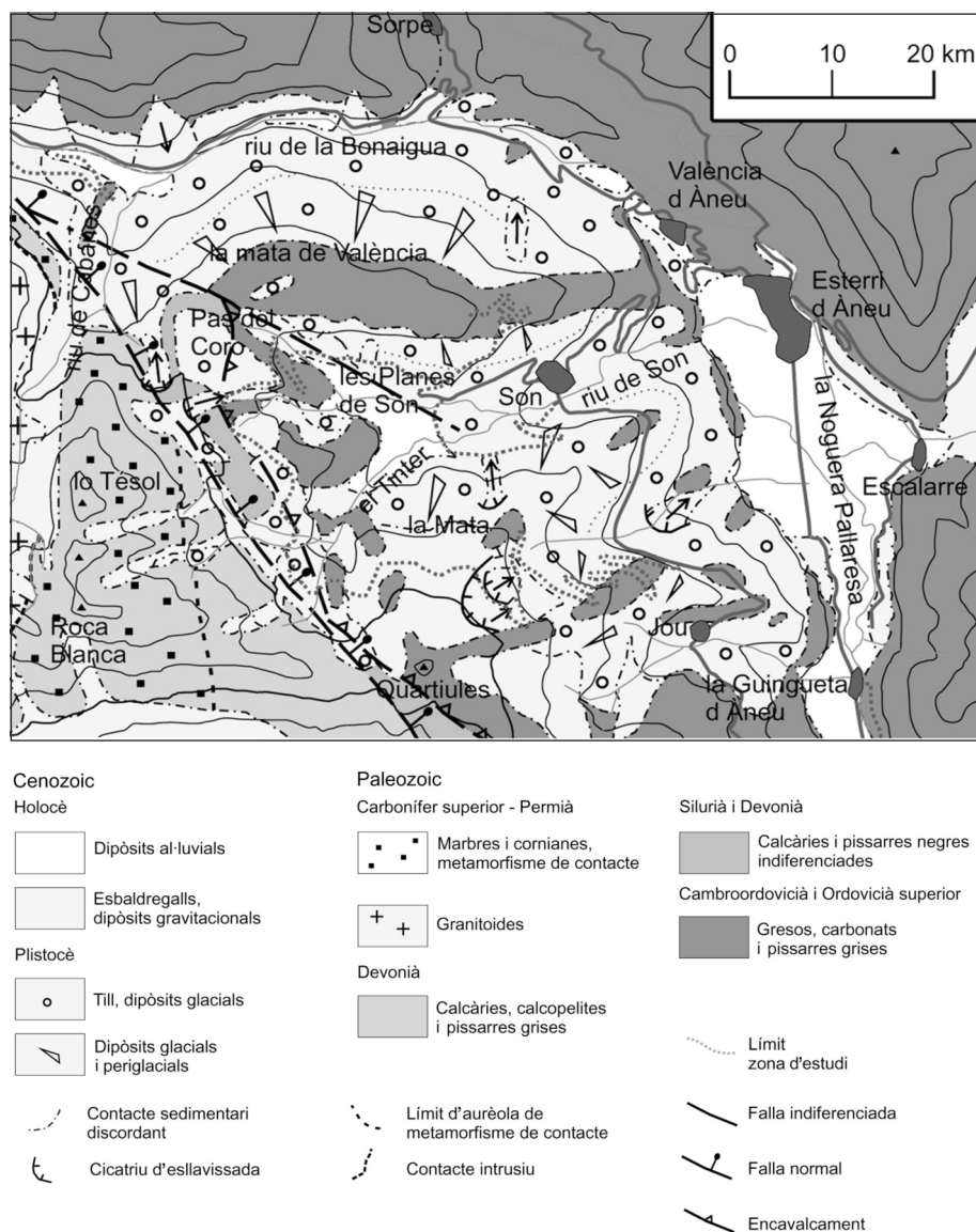
FIGURA 4. Esquema geològic simplificat de la zona de les Planes de Son i la mata de València. Reflecteix la distribució cartogràfica dels diversos materials que afloren a la zona d'estudi i als voltants.
