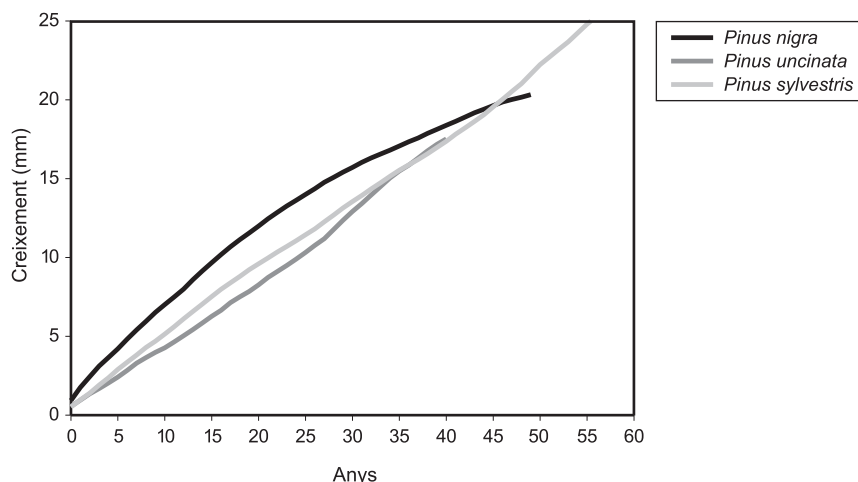
FIGURA 14. Corbes de creixement diametral per espècie. La gràfica correspon a la mitjana dels creixements per a cada edat dels diferents arbres mesurats. Si el nombre de mostres per a una edat determinada és menor de cinc, no es donen els valors.
